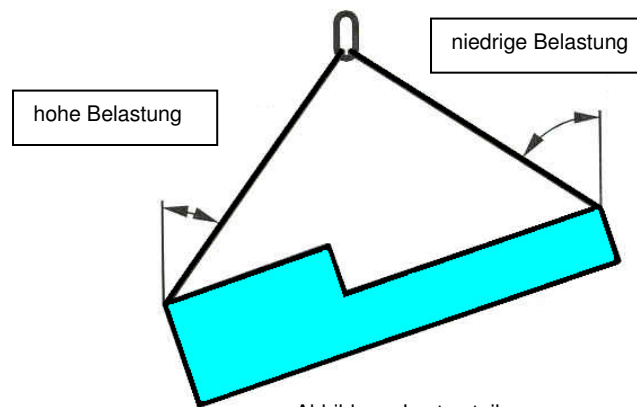
Abbildung: Lastverteilung
