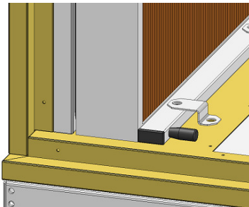
Abbildung: Klemmschienenfilter
