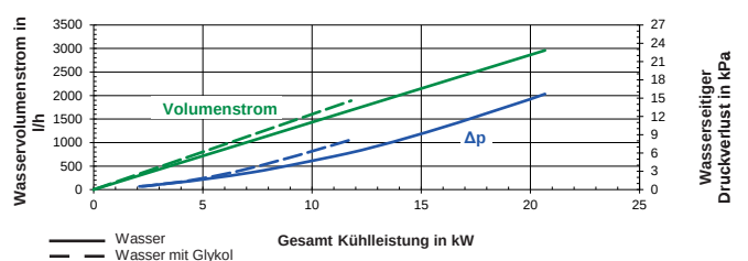
Wasservolumenstrom und wasserseitiger Druckverlust
